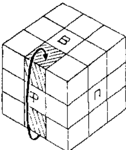
A10 L^{-1}P\phi^2L^{-1}P^{-1}H^2 \phi n \rightarrow \phi \delta
