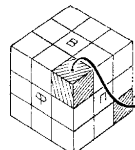
A8 FH^2F^{-1}H^{-1} \phi \delta n \rightarrow n \tau
