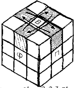
A4 F^{-1}B(P^2B^2)^3B^{-1}F^{-1} \begin{cases} \delta l \leftrightarrow \delta n \\ \delta \phi \rightarrow \delta \tau \end{cases}
