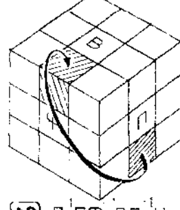
A9 L^{-1}PH^{-1}LPH n n \rightarrow \phi \delta
