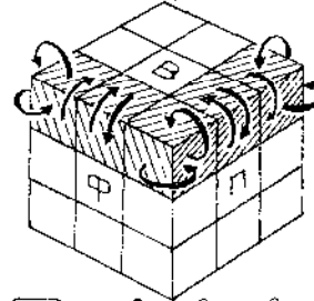
A12 FV\phi^2L\phi L^2V\phi V^2 \begin{cases} \phi \delta l \rightarrow \phi \delta n \rightarrow \phi \delta n \rightarrow \phi \delta l \\ \phi \delta n \rightarrow \phi \delta n \rightarrow \phi \delta n \rightarrow \phi \delta n \\ n \tau \delta \rightarrow n \tau \delta \rightarrow n \tau \delta \rightarrow n \tau \delta \\ \phi \delta \rightarrow \phi \delta \rightarrow \phi \delta \\ n \delta \rightarrow n \delta \rightarrow n \delta \end{cases}
