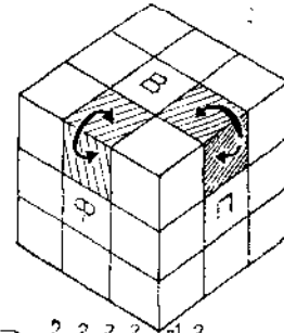
A6 P^2\phi P^2\phi^{-1}B^{-1}PB\phi B\phi^{-1} \phi B \rightarrow \phi \delta
