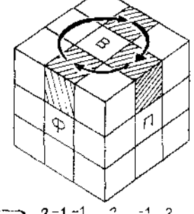
A11 P^2H^{-1}L^{-1}PB^2LP^{-1}\phi^2HH^2 \begin{cases} \phi \delta \rightarrow \tau \delta \rightarrow n \delta \rightarrow \phi \delta \\ \phi \delta \rightarrow \tau \delta \rightarrow n \delta \rightarrow \phi \delta \end{cases}
