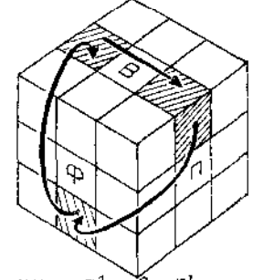
A5 B^{-1}PLF^2PL^{-1}B \begin{cases} \phi n \rightarrow \delta l \rightarrow \delta n \\ \delta n \rightarrow \phi n \end{cases}
