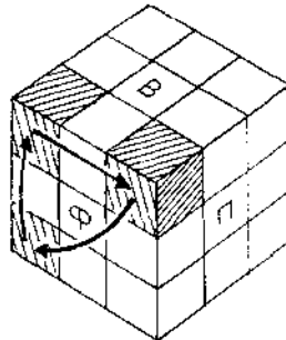
A7 L^{-1}B^{-1}P^{-1}B^{-1}PB \phi \delta l \rightarrow \phi \delta n \rightarrow \phi l n \rightarrow \phi \delta l
